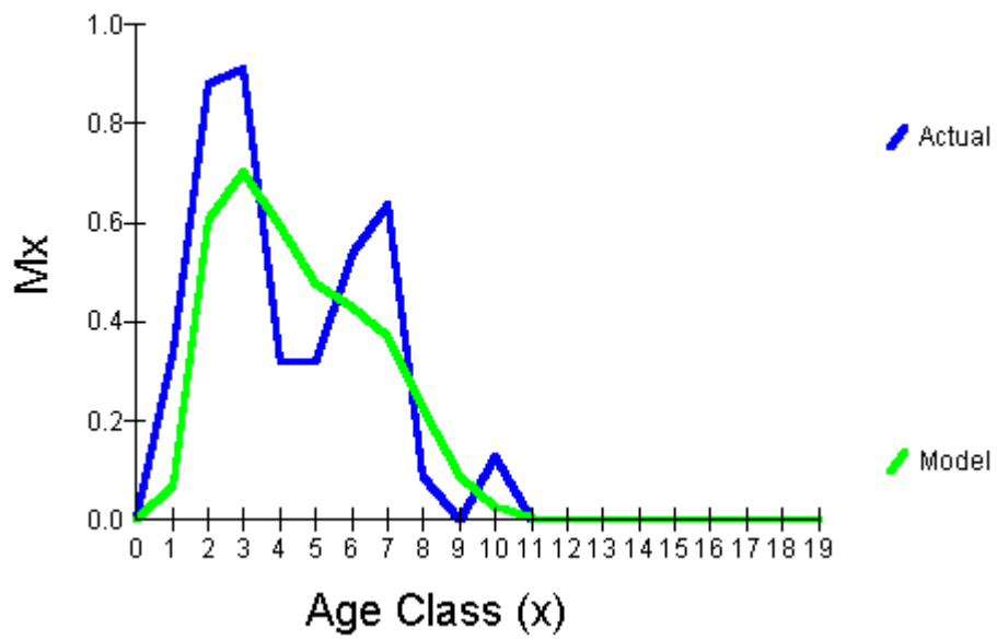
Mx - Actual vs Model - Males
