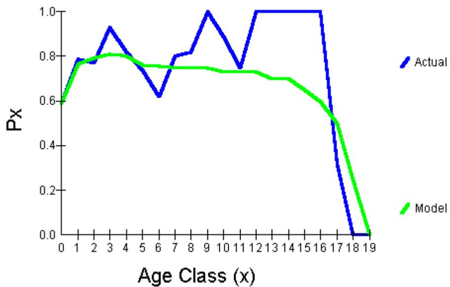
P_x - Actual vs Model - Females
