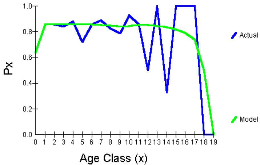
P_x - Actual vs Model - Males
