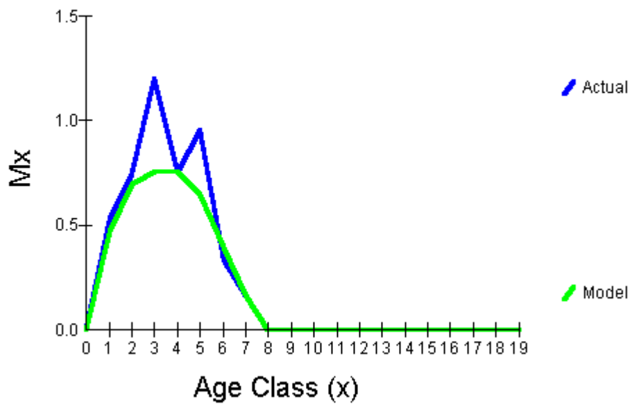
Mx - Actual vs Model - Females
